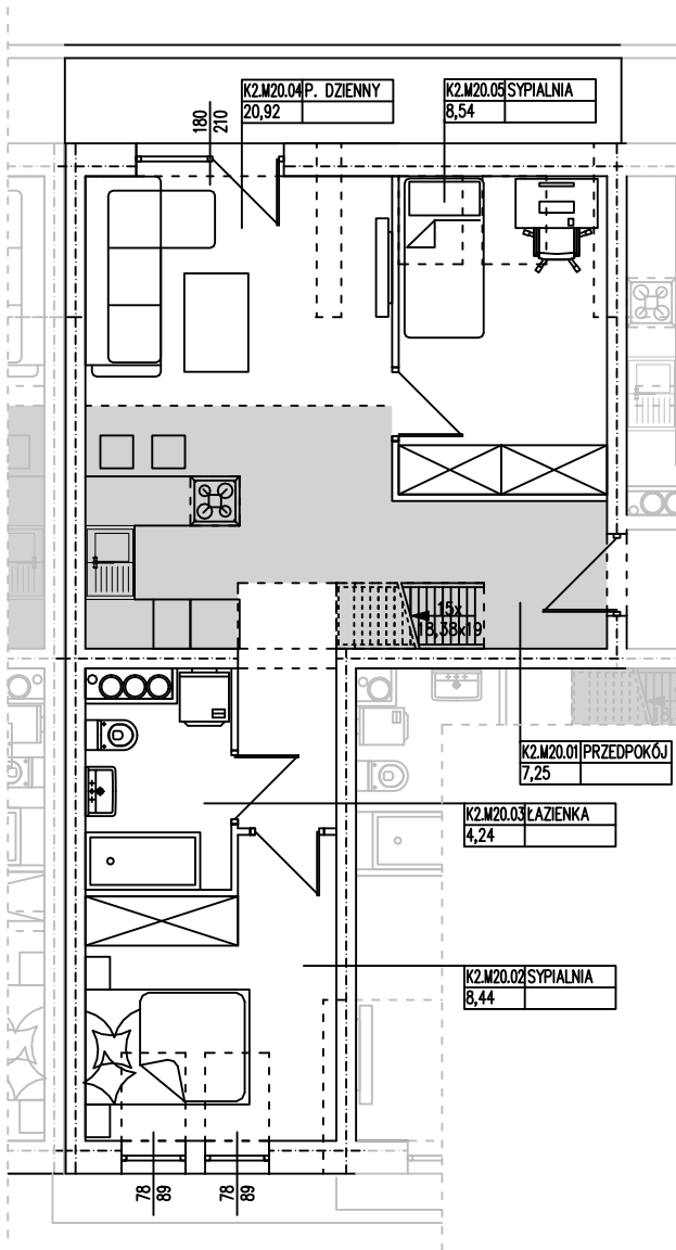
RZUT III PIĘTRA
