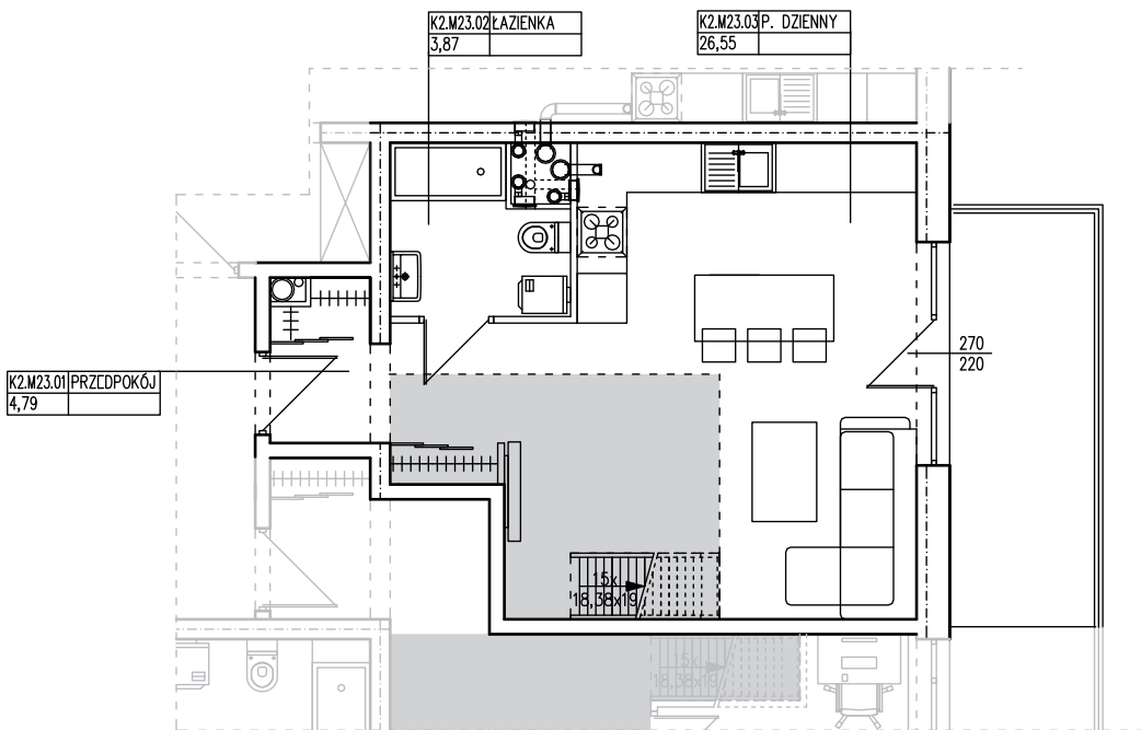
RZUT III PIĘTRA
