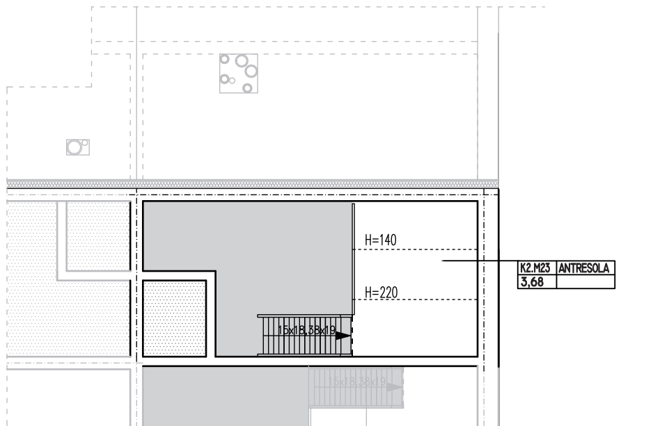
RZUT ANTRESOLI III PIĘTRA
