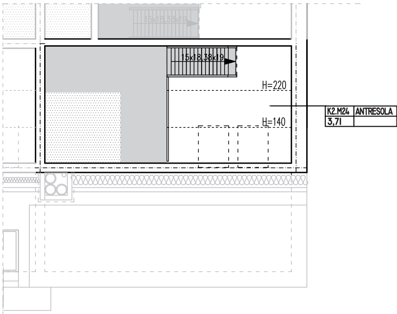
RZUT ANTRESOLI III PIĘTRA
