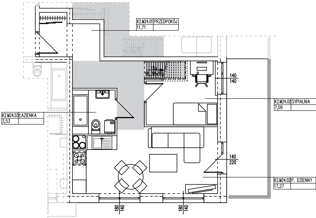
RZUT III PIĘTRA
