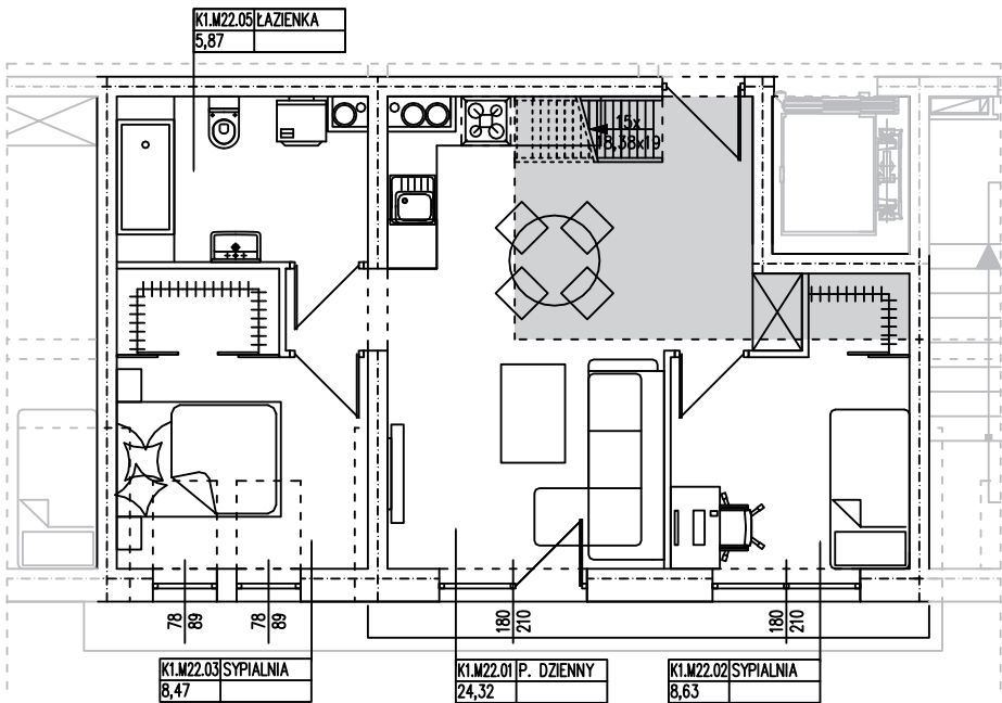
RZUT III PIĘTRA
