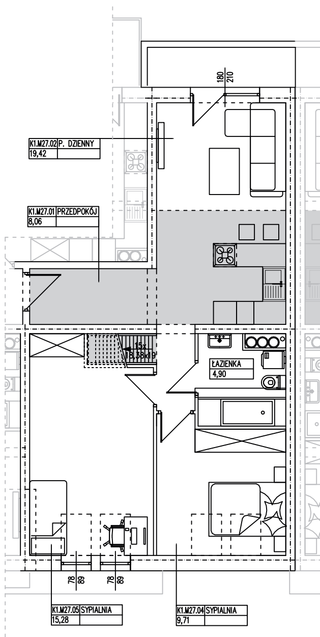
RZUT III PIĘTRA
